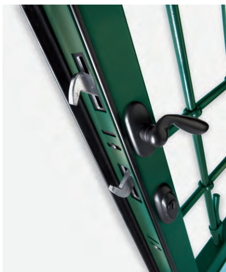
Serratura a doppio gancio per Grata a battente
